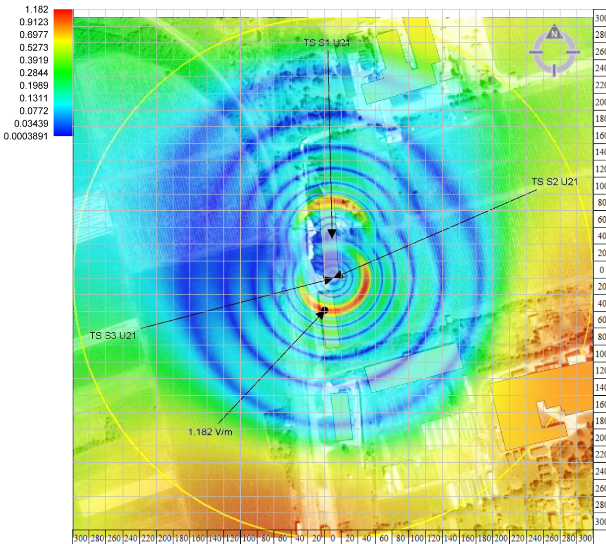
Slika 6.9. Jačina električnog polja radio-sistema UMTS2100 na nivou 1,5 m
