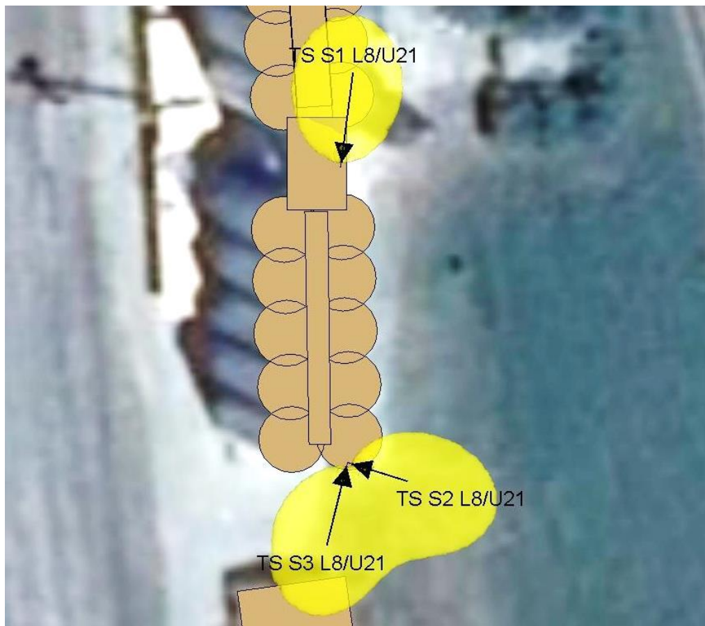
Slika 6.4 Prikaz polja koje stvaraju antene pri maksimalnom opterećenju, pogled iz perspektive
