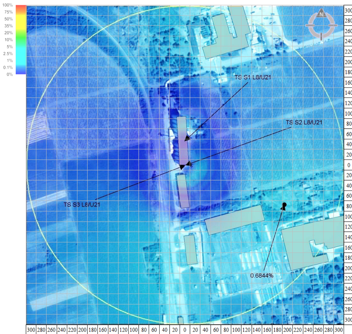
Slika 6.10. Izloženost od radio-sistema UMTS2100 i LTE800 operatora “Telekom Srbija” na nivou 1,5 m
