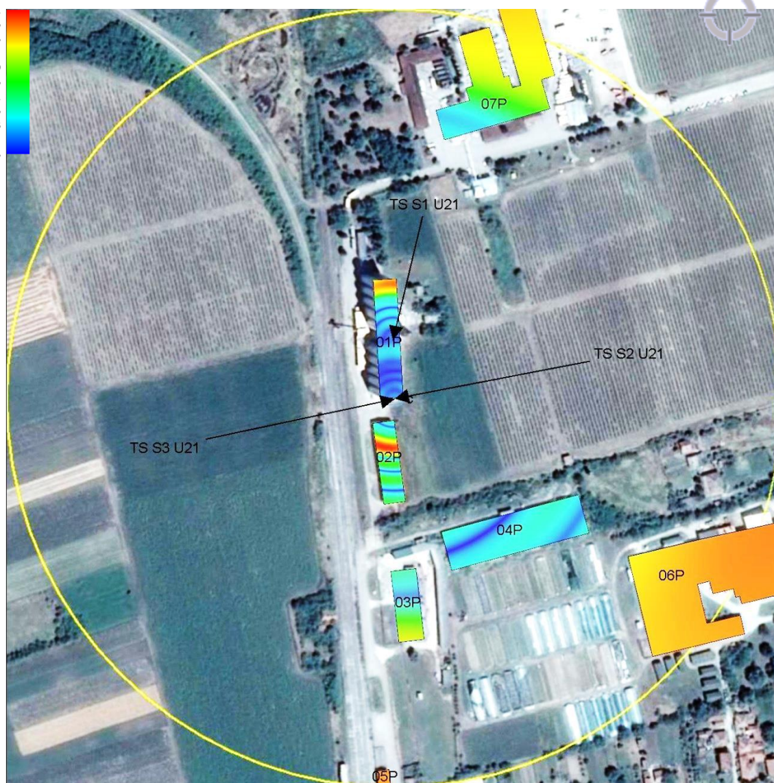
Slika 6.11. Jačina električnog polja radio-sistema UMTS2100 na nivoima najizloženijih spratova
